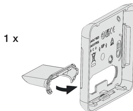
Rückseitige Abdeckung und Ständer für Tischaufstellung
